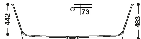
Schnitt-vorne
