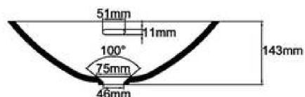
Schnitt-Vorne
